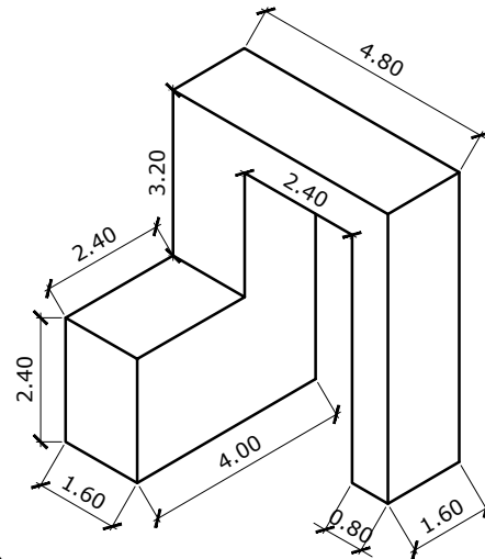
Isometrico 2
